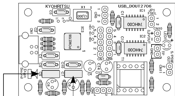
C5 フィルムコンデンサ 0.022 \mu F C7 フィルムコンデンサ 0.022 \mu F(223)
