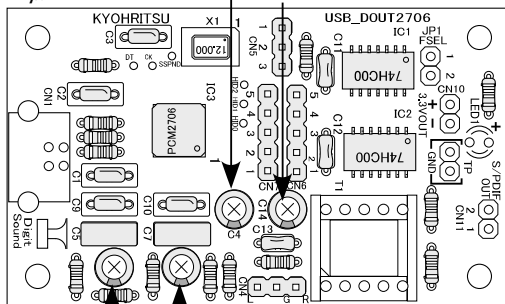
C6 電解コンデンサ 16V 100 \mu F C8 電解コンデンサ 16V 100 \mu F
