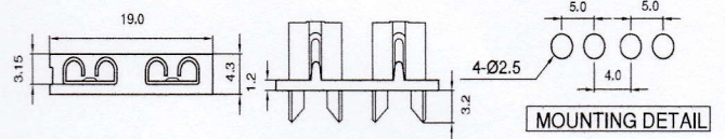
CQ-122 For AST Mini Blade Type Fuse
