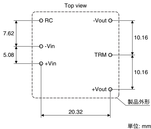
図8-1 基板取付け寸法図
