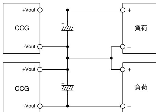
図6-9 土出力使用の直列運転
