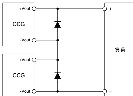
図6-8 出力電圧積み重ね直列運転
