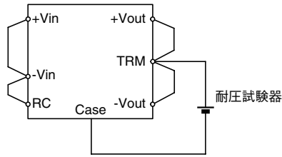
図6-12 出力-ケース間耐電圧試験方法
