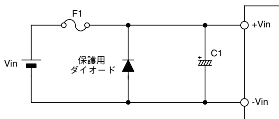
図5-2 入力の逆接続保護
