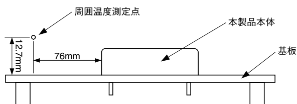
図7-1 周囲温度に対する出力ディレーティングの測定方法(自然空冷の場合)
