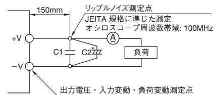
特性測定回路
