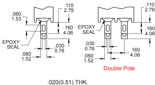
M1 Solder lug
