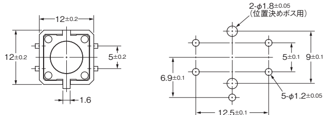
プリント基板加工寸法(参考) (TOP VIEW) (プリント基板厚 t=1.6)
