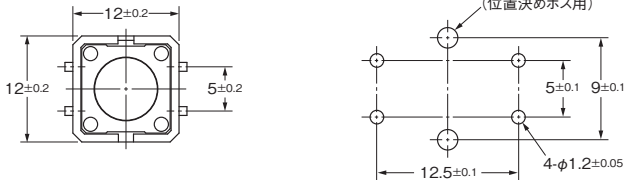
プリント基板加工寸法(参考) (TOP VIEW) (プリント基板厚 t=1.6)
