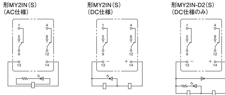
端子配置/内部接続図(BOTTOM VIEW)
