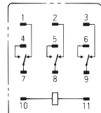
端子配置/内部接続図 (BOTTOM VIEW) 基準形
