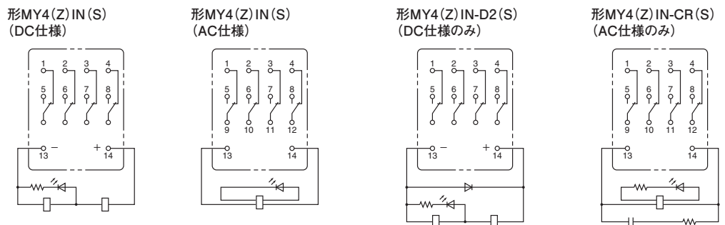
端子配置/内部接続図(BOTTOM VIEW)
