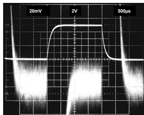
図 32.大信号パルス応答とセトリング・タイム G = -1000 ( 5 \text{ mV} = 0.01\% )、 C_L = 100 \text{ pF}
