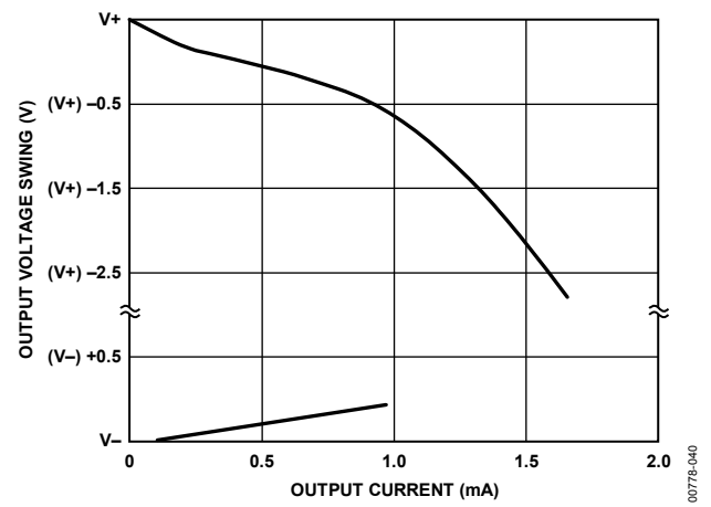
図 40. 出力電流対出力電圧振幅
