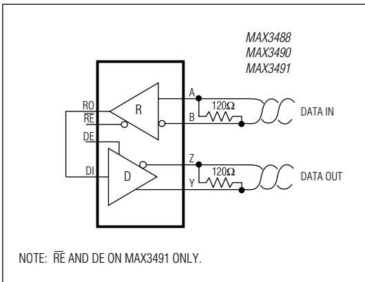
図23. MAX3488/MAX3490/MAX3491のシングルラインリピータ
