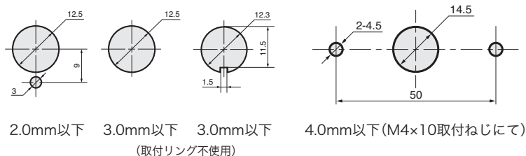
取付穴寸法図・取付パネル有効板厚
