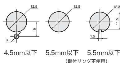
取付穴寸法図・取付パネル有効板厚
