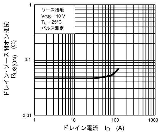
図 8.6 R_{DS(ON)} - I_D
