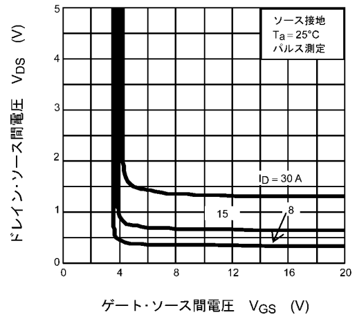
図 8.4 V_{DS} - V_{GS}
