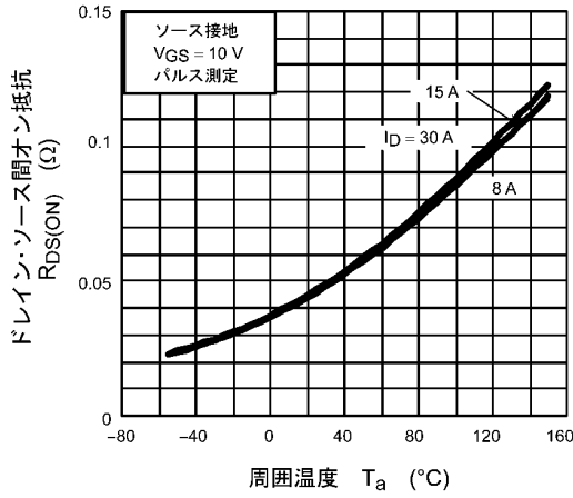
図 8.7 R_{DS(ON)} - T_a
