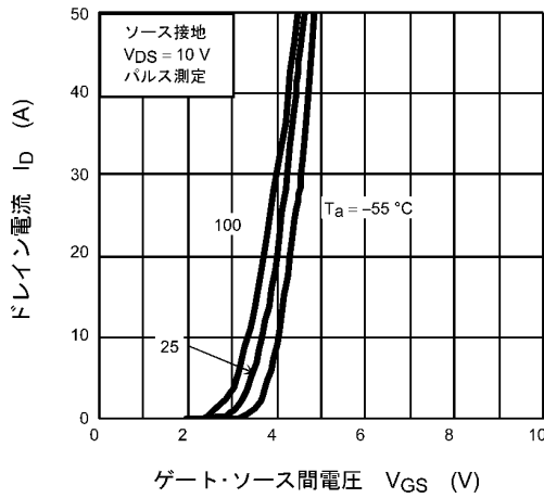
図 8.3 I_D - V_{GS}
