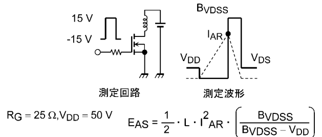
図 8.16 測定回路/測定波形
