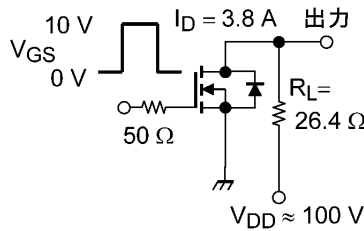
図 6.2.1 スイッチング時間の測定回路例
