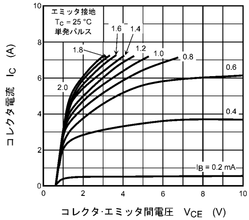
図 7.2 I_C - V_{CE}
