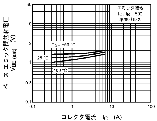
図 7.6 V_{BE(sat)} - I_C
