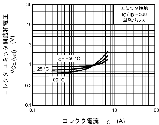
図 7.5 V_{CE(sat)} - I_C
