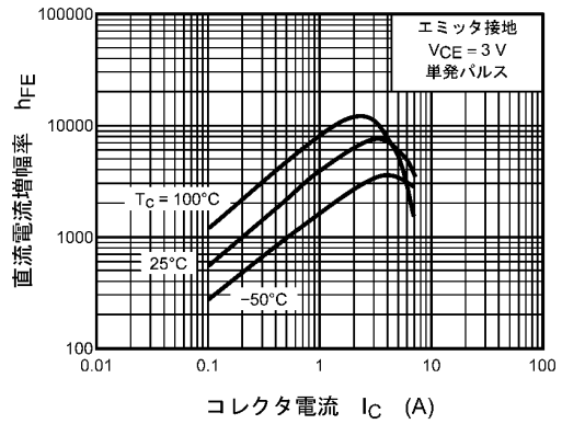
図 7.4 h_{FE} - I_C
