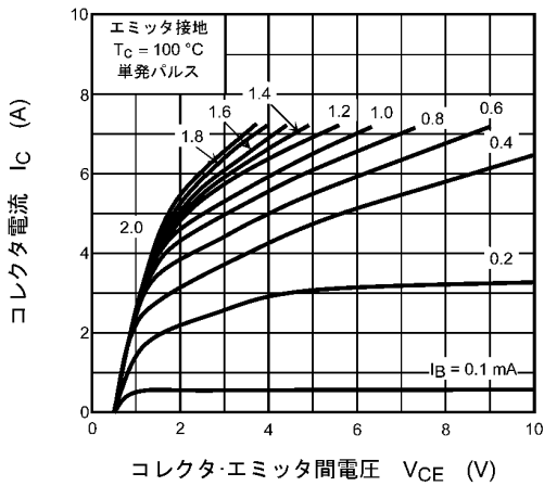
図 7.3 I_C - V_{CE}
