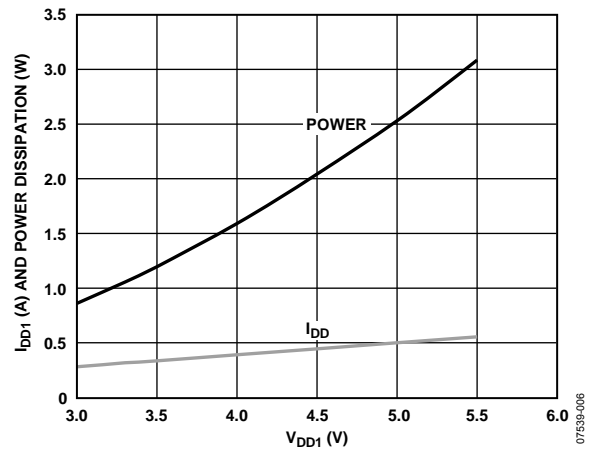
図 7. V_{DD1} 電源電圧対短絡入力電流および消費電力
