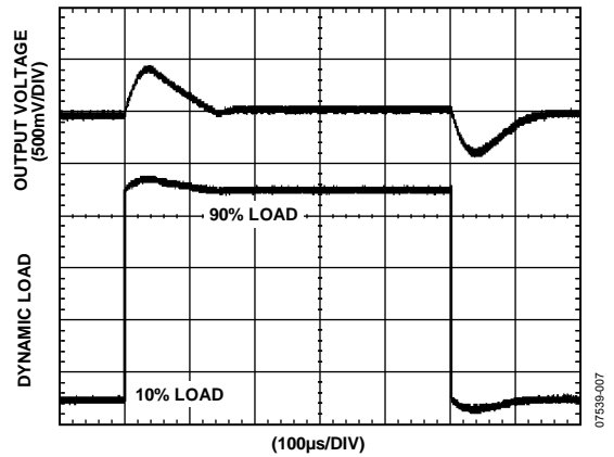
図 8. V_{ISO} 過渡負荷応答 5 V 出力、10%→90%の負荷ステップ
