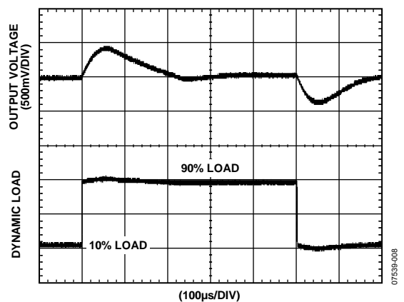
図 9. V_{ISO} 過渡負荷応答 3 V 出力、10%→90%の負荷ステップ
