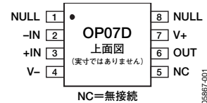
図1. 8ピンSOIC_N (R-8)、8ピンDIP (N-8)
