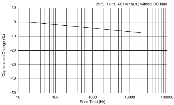
静電容量-経時変化
