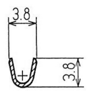
B-B 断面
