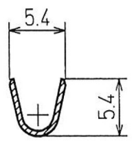
A-A 断面
