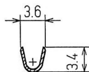
断面B-B
