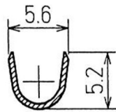
断面A-A
