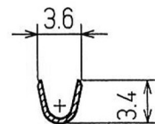
断面B-B
