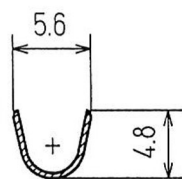
断面A-A
