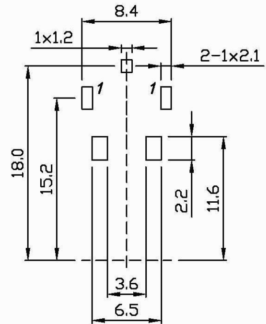
P.C.B LAYOUT(±0.1) (BOTTOM VIEW)
