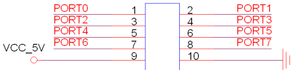
図 5. ポートコネクタピン番号
