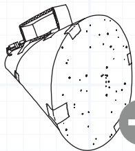
p22 星図
