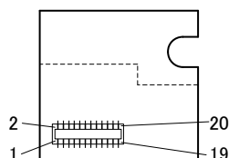
図 3 IMBLE 端子配置図
