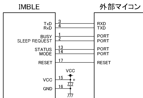
図2 外部マイコンとの接続例
