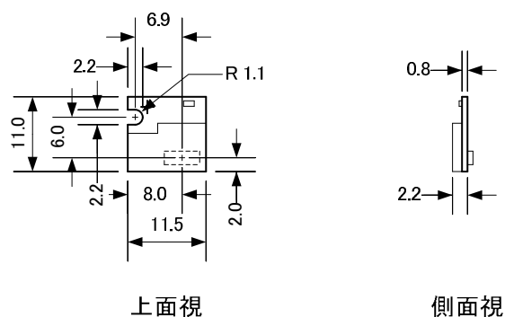
図4 外形寸法図
