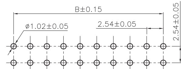
P.C.B. Layout
