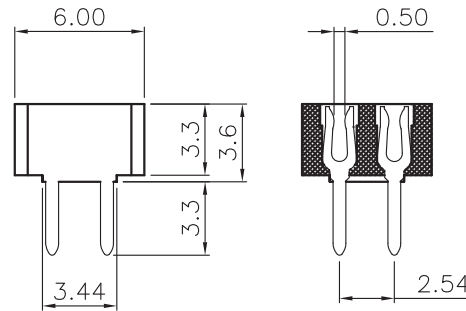
SECTION B-B 1:1
