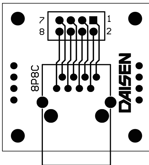
MJ8配線図 (Top View)
