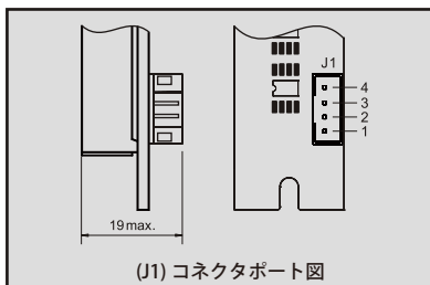
配線図 (J1)
