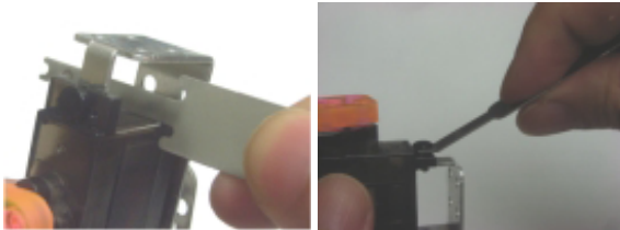
■リベットリムーバー使用例
